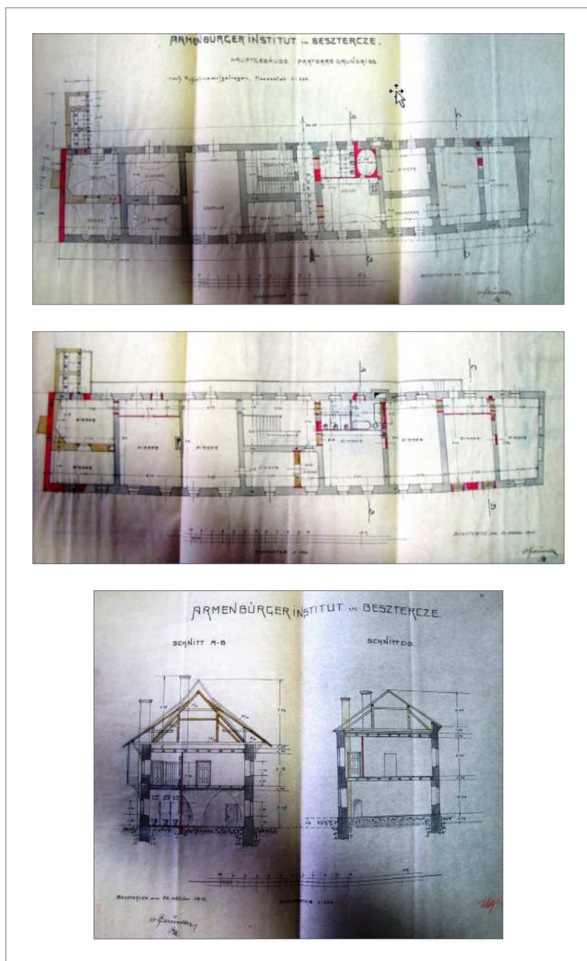
Pl. XV. Plan și secțiune a Armemburger Institut (Căminul pentru persoane vârstnice) realizat de către arhitectul Otto Dahinten (1916), Arhivele Naționale Bistrița, Fond Primăria Bistrița, dosar 512.
